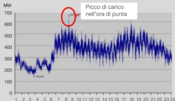
1 giorno FFS (16,7 Hz)
